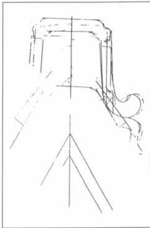
▲鬼板の原寸引付け図
