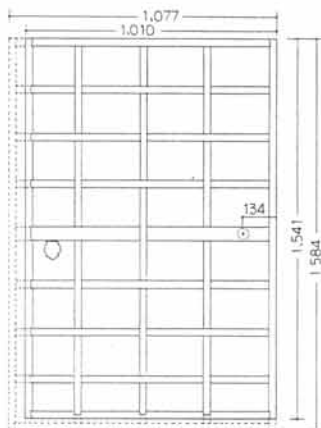
図1 襖障子骨組 (点線部分は復原)
