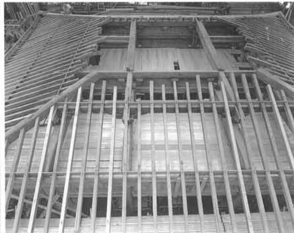
組立中－化粧垂木の状況
