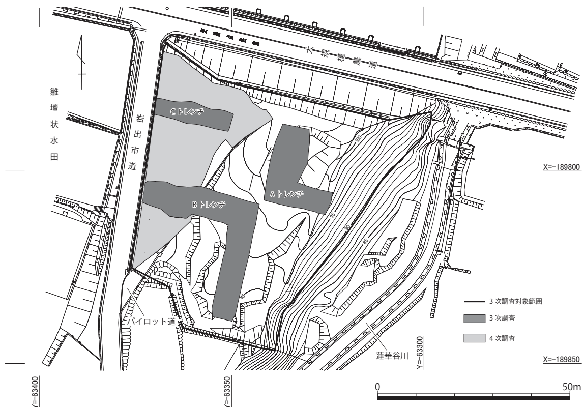
第13図 3次調査・4次調査 調査区位置図 (S=1:1,000)
