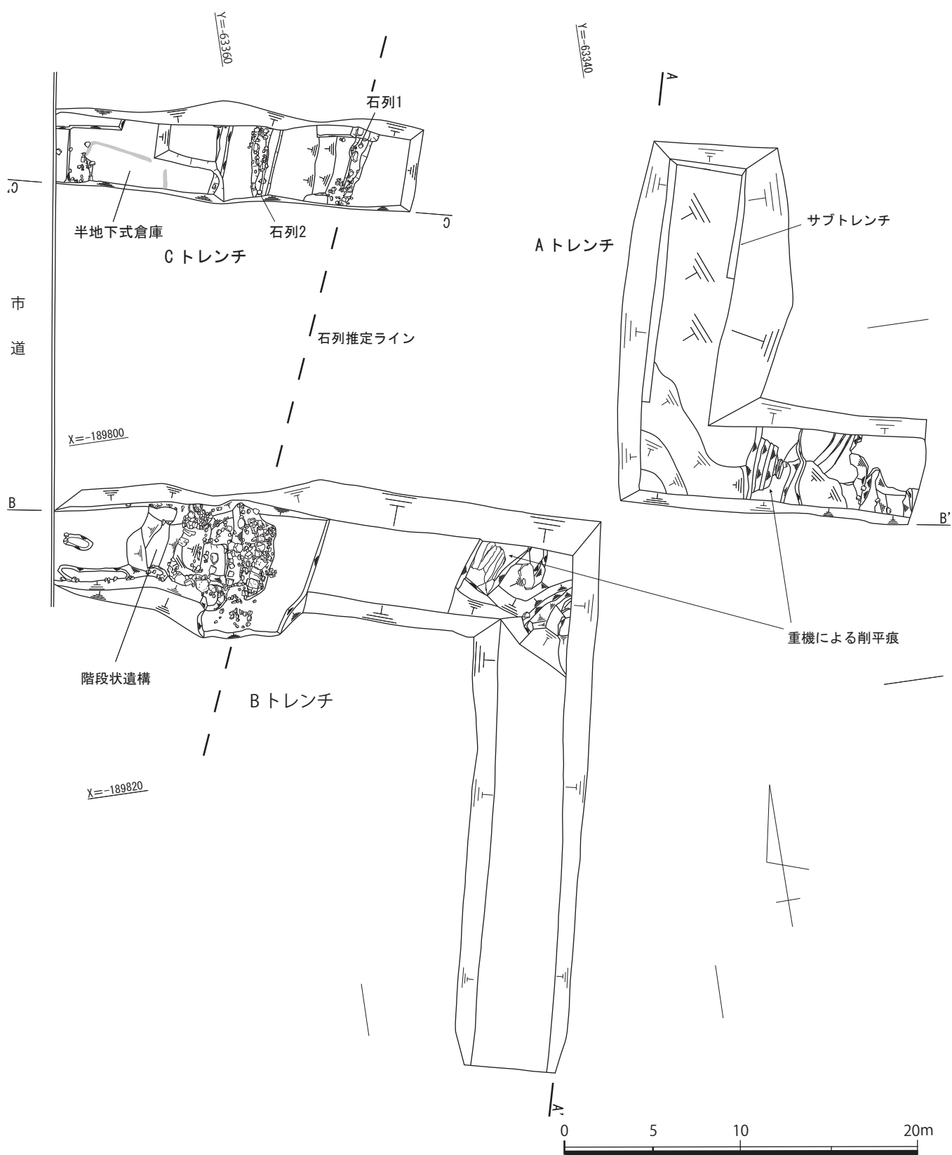
第14図 3次調査遺構平面図 (S=1/300)
