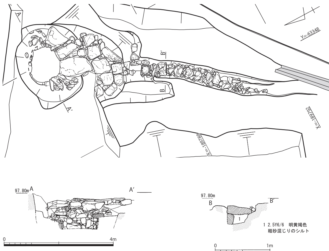
第18図 井戸・溝6 平面図及び井戸立面図 (S=1/80)、溝6断面土層図 (S=1/40)
