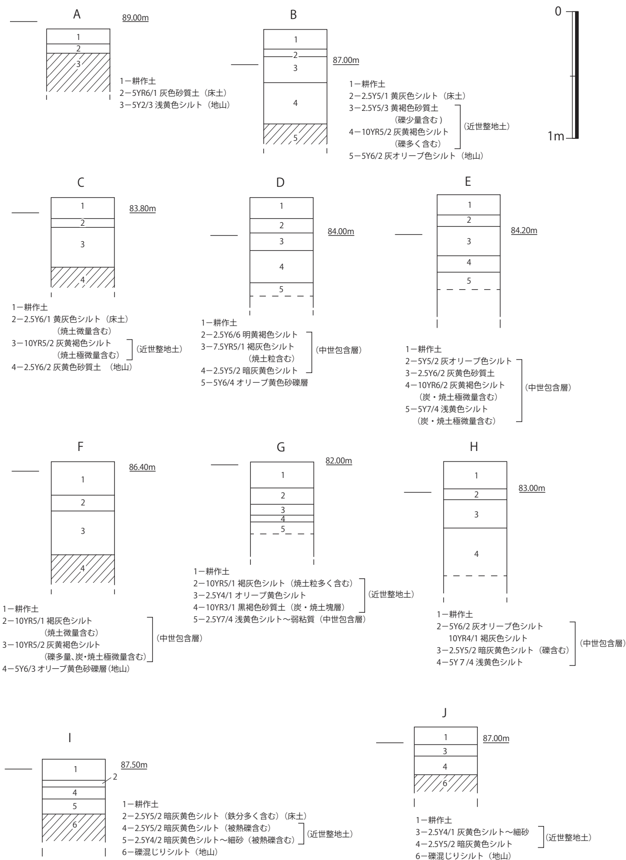
第 5 図 1 次調査・2 次調査土層柱状図 (S=1/30)
