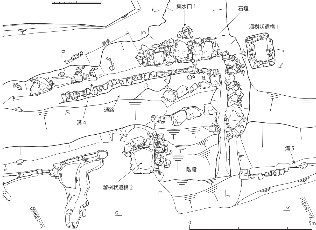
第22図 階段・石垣・集水口1・溜樹状遺構1・溜樹状遺構2・溝4平面図及び石垣立面図(S=1/80) 溜樹状遺構1土層断面図(S=1/40)
