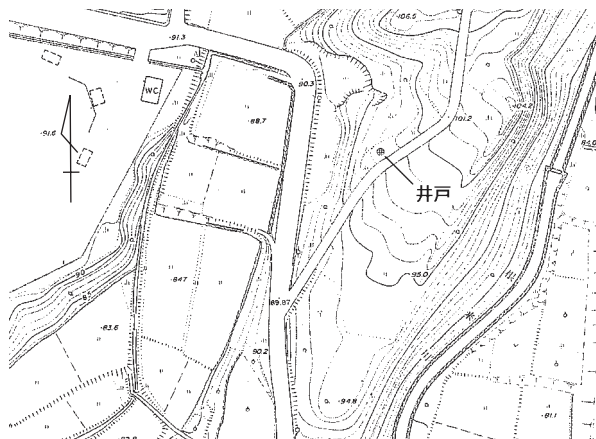
第17図 昭和55年測図の地形図 (S=1/3,000)
