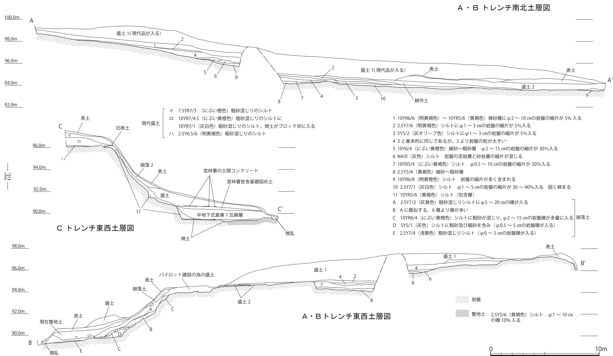
第15図 3次調査 A・B トレンチ南北及び東西土層図、C トレンチ東西土層図 (S=1/200)
