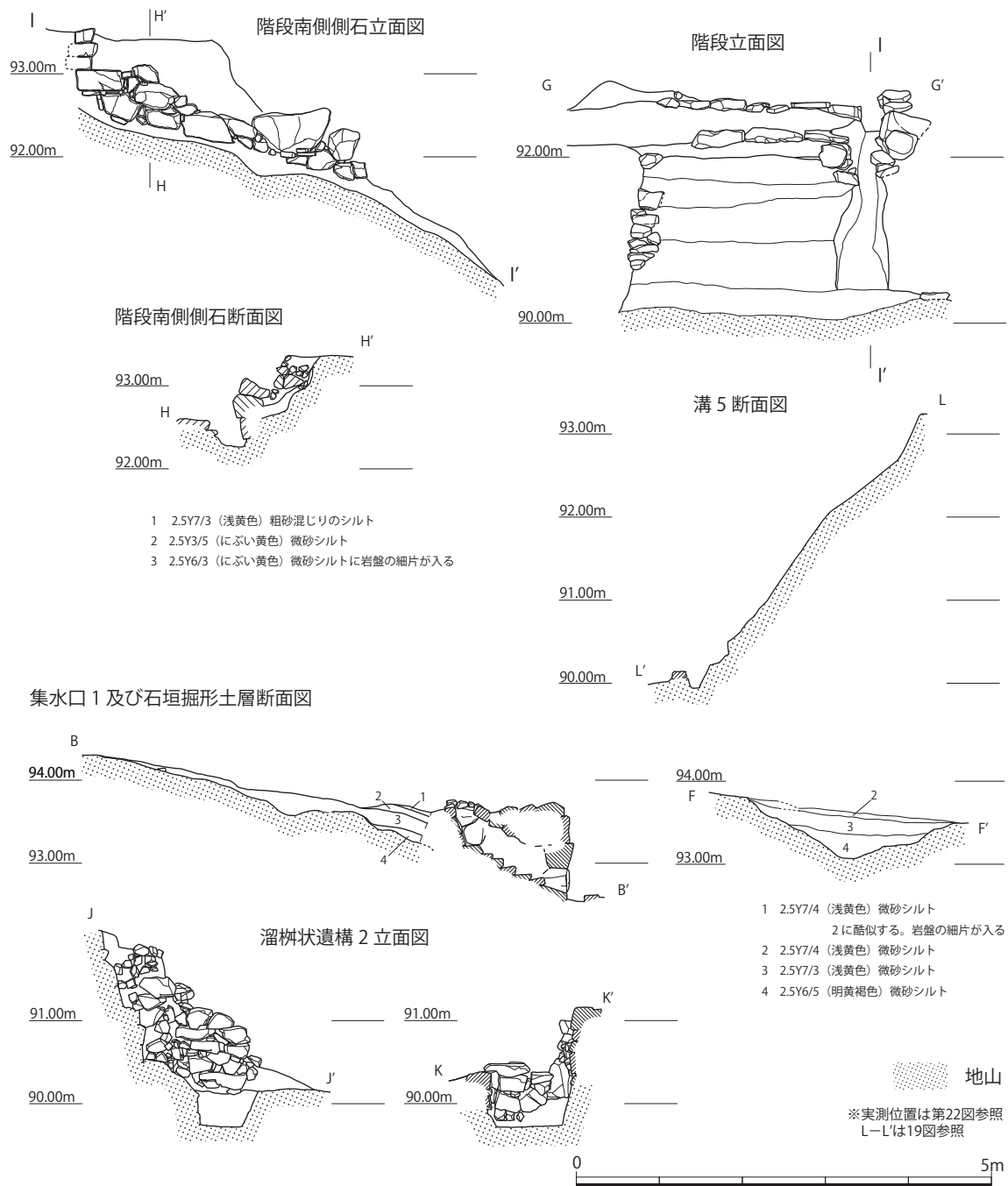
第23図 階段・階段南側石・溜樹状遺構 2 立面図、集水口 1 及び石垣掘形・階段南側石・溝 5 断面図 (S=1/80)
