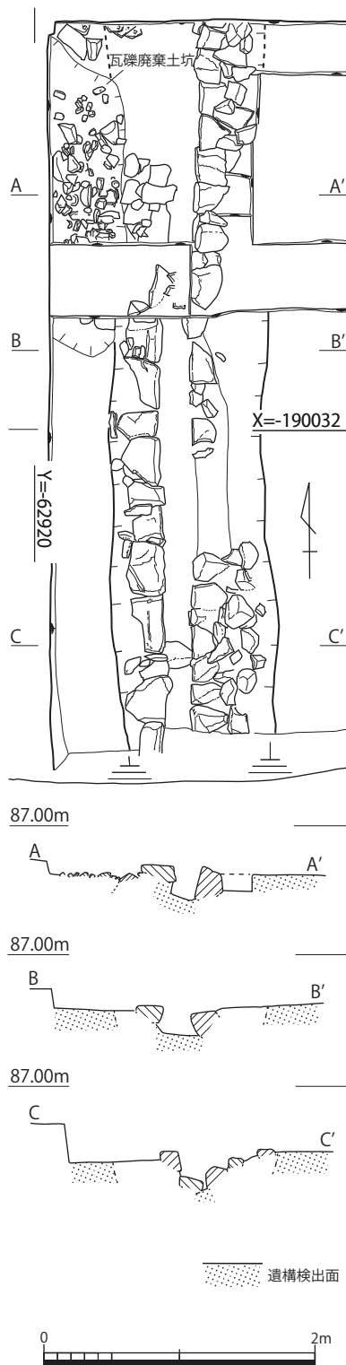
第11図 J区遺構44 平面図及び断面図 (S=1/50)
