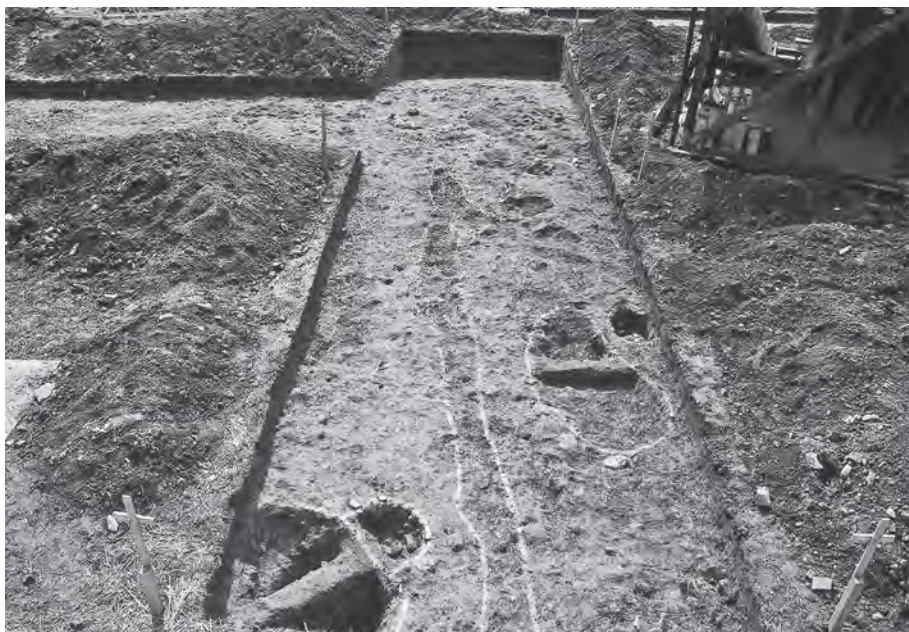
3 B区 遺構 7 土坑・8 土坑・9 溝 検出状況 (北から)
