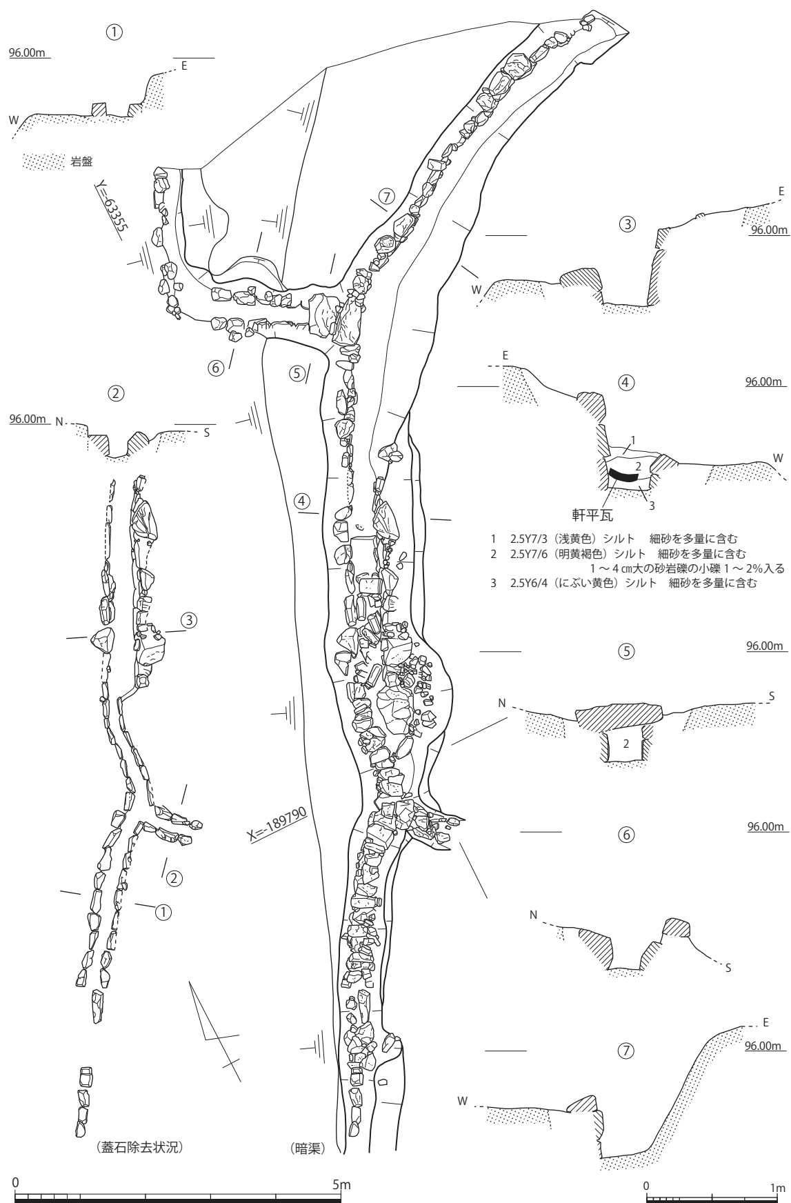
第 20 図 溝 1 平面図 (S=1/80) 及び土層図・断面図 (S=1/40)
