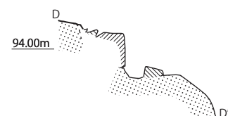
溝4断面図
