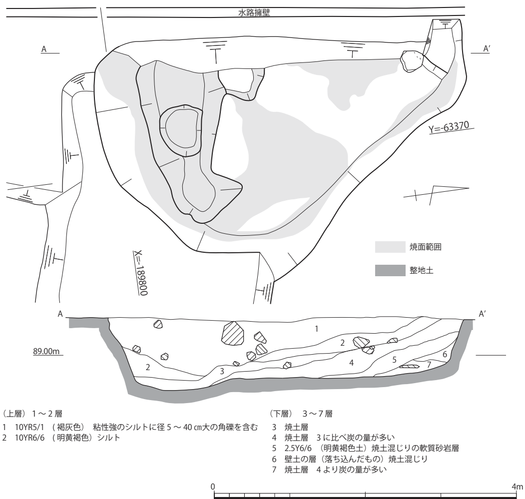
第26図 半地下式倉庫2 平面図及び土層図 (S=1/50)
