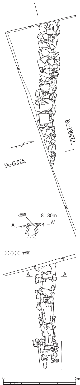
第 8 図 G 区遺構 30 平面図及び断面図 (S=1/50)
