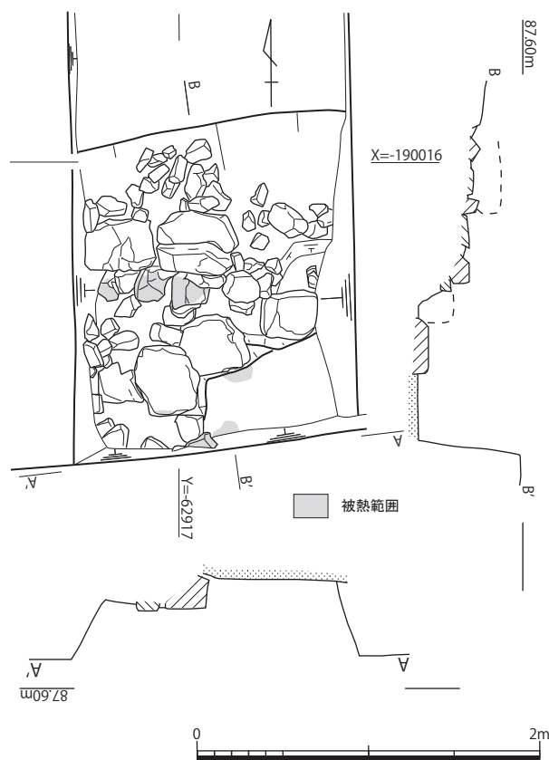
第9図 I区階段状遺構 平面図及び断面図 (S=1/40)
