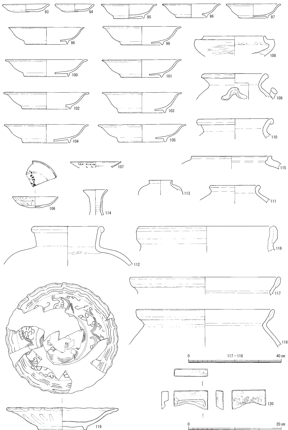
第 29 図 半地下式倉庫 3 出土遺物実測図 1
