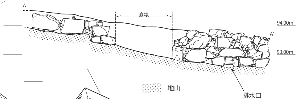
石垣立面図
