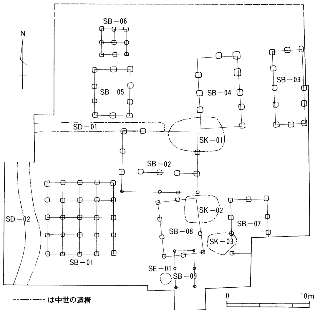
図15 主要遺構配置図
