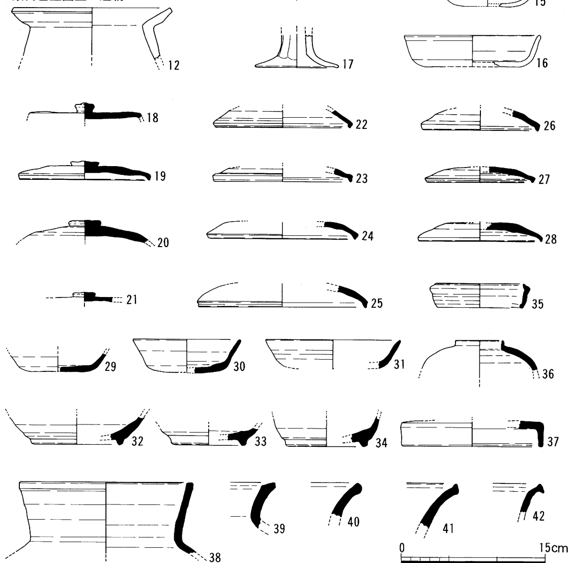
図12 遺物実測図(1)
