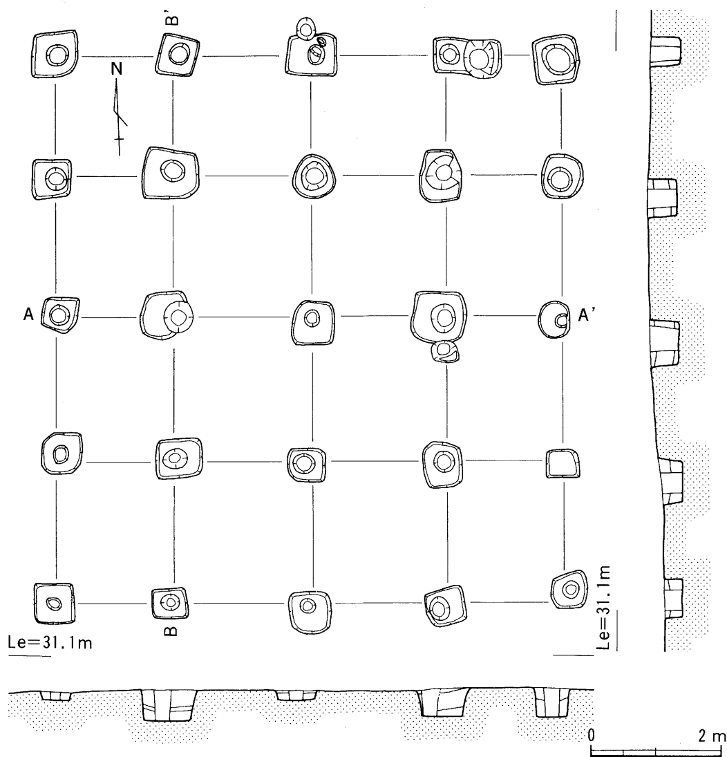
図4 SB-01 実測図
