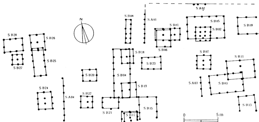
図17 栗島遺跡A区遺構配置図
