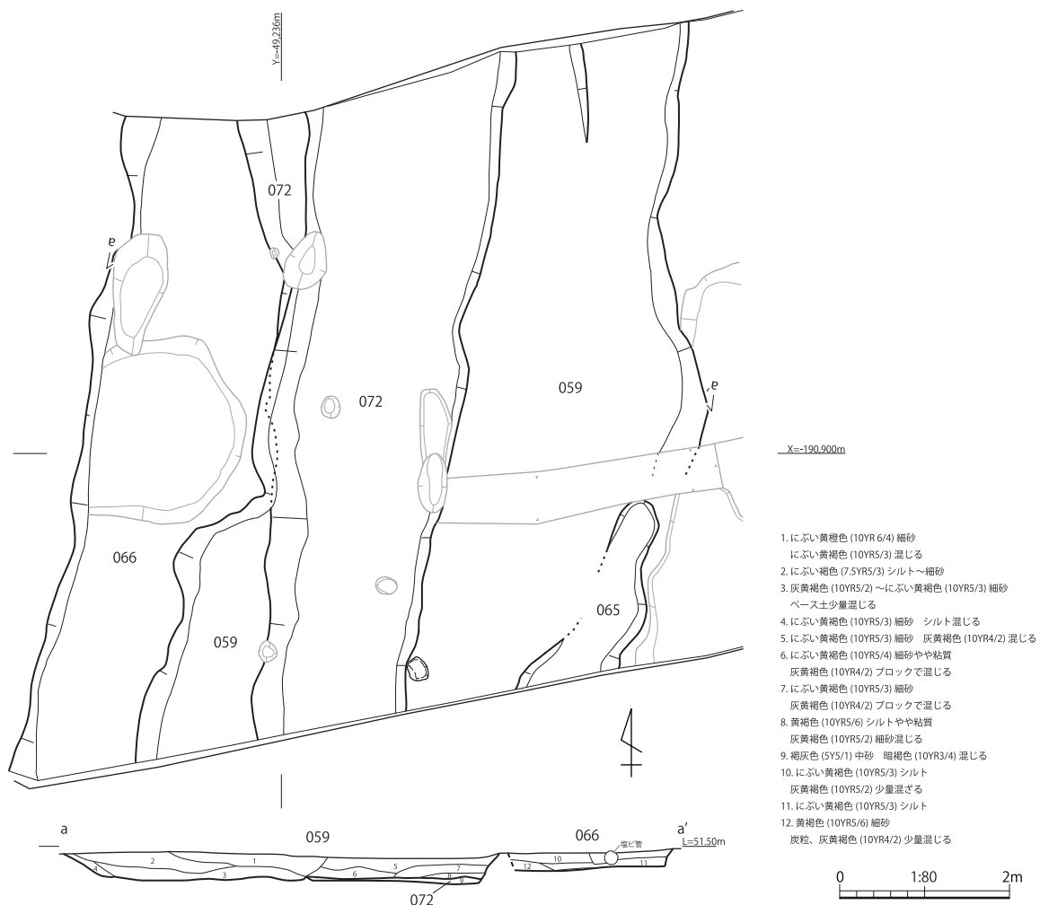
図7 066・059・072 溝平面図・断面図
