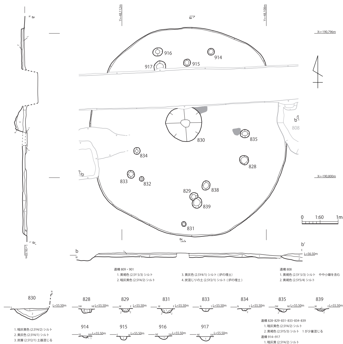
図18 809 竪穴住居平面図・断面土層図
