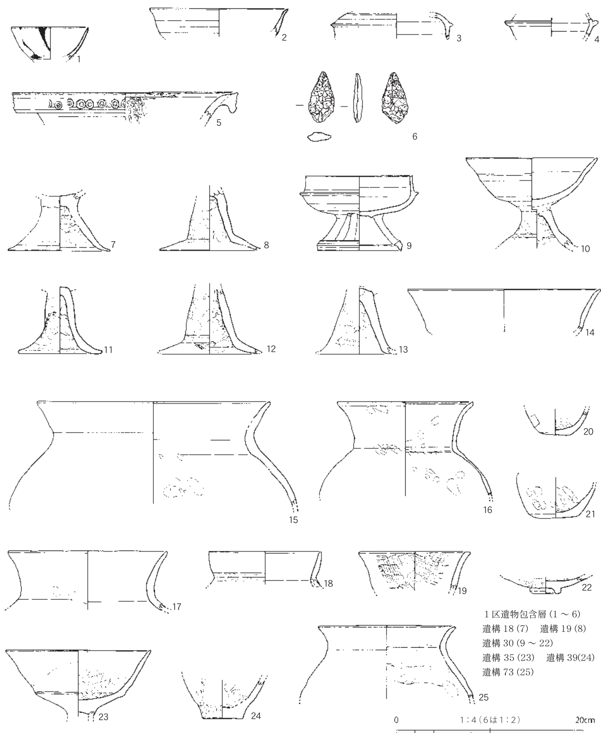
図8 西沢田遺跡出土遺物実測図 (1)
