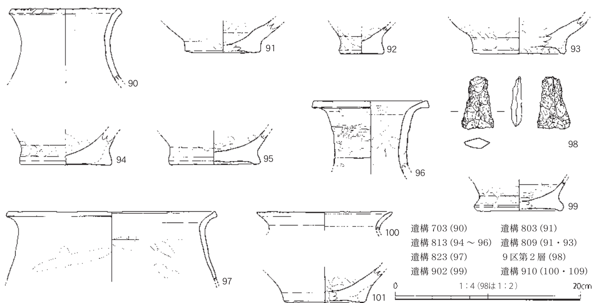
図21 東浜田遺跡出土遺物実測図(3)
