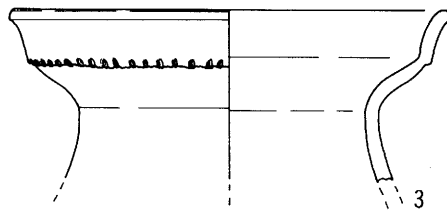
圖 4 遺物實測圖 1
