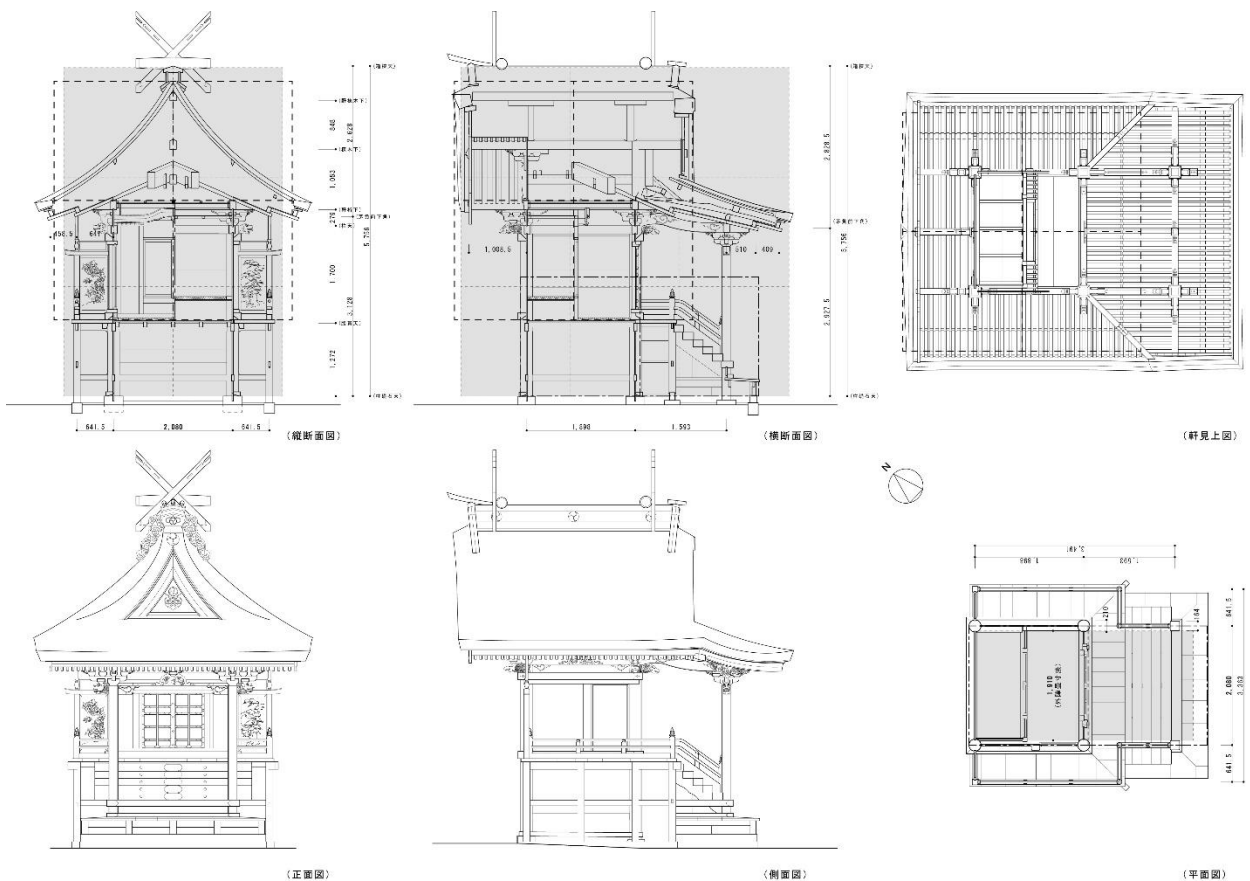
図1 須賀神社本殿(第一殿)での基本図面作成と基幹寸法等計画性の検討状況 → 図中の網掛は畳の長手寸法を一边とした正方形グリッドを、破線2種は身舎正面の柱間真々寸法を一边とした正方形グリッドを表現したもの。 → 本殿の大きさは、平面(畳4枚分)、正面(畳12枚分)、側面(畳18枚分)と畳の寸法を基準として設定されたことがうかがえる。
